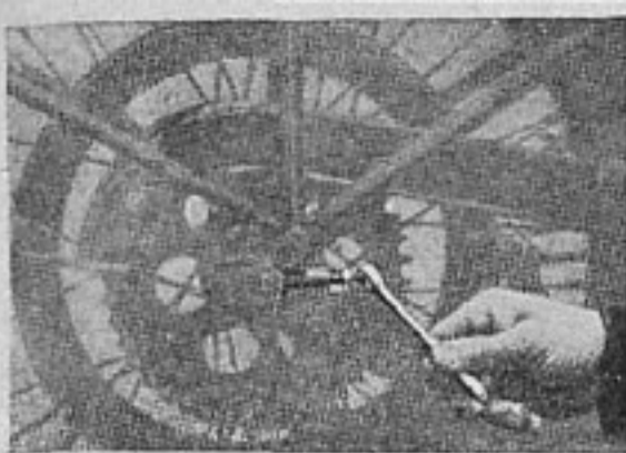
Регулировка натяжения задней цепи путем подворачивания регулирующих натяжек
