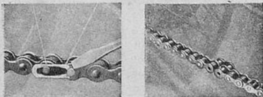
Слева — снятие пружины замочного звена при помощи отвертки. Справа — раз'единение цепи после снятия пружины и боковинки замочного звена
