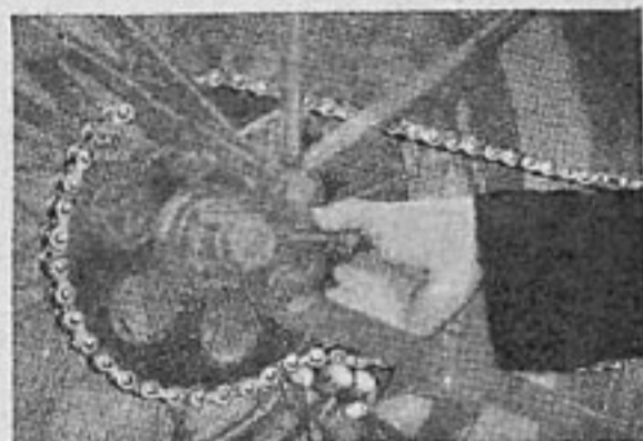
Способ испытания задней цепи на нормальный провес. Цепь требует подтяжки, если к шестерне можно прижать, кроме нормально находящихся в сцеплении с ней, три или более звена
